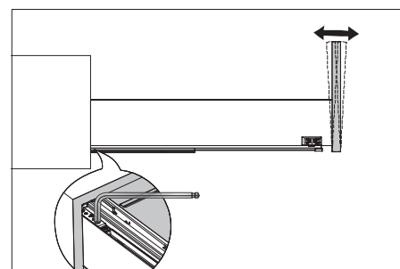
Ajuste tilt(atraves da chave allen)
