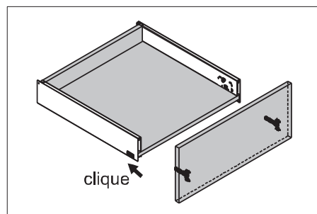
Montagem de frente
