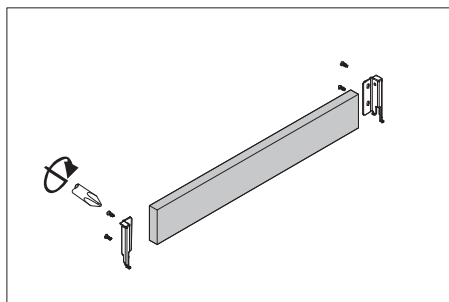
Montagem de traseiro
