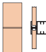
Travessa aparente
